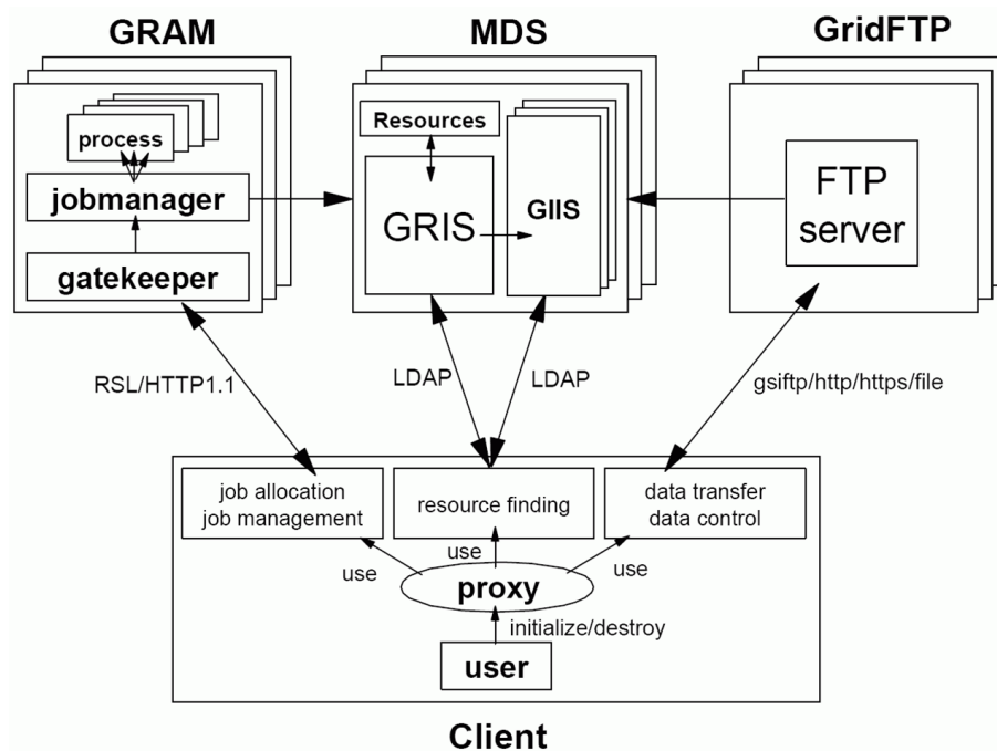
Figura 3.4. Globus:Main components
