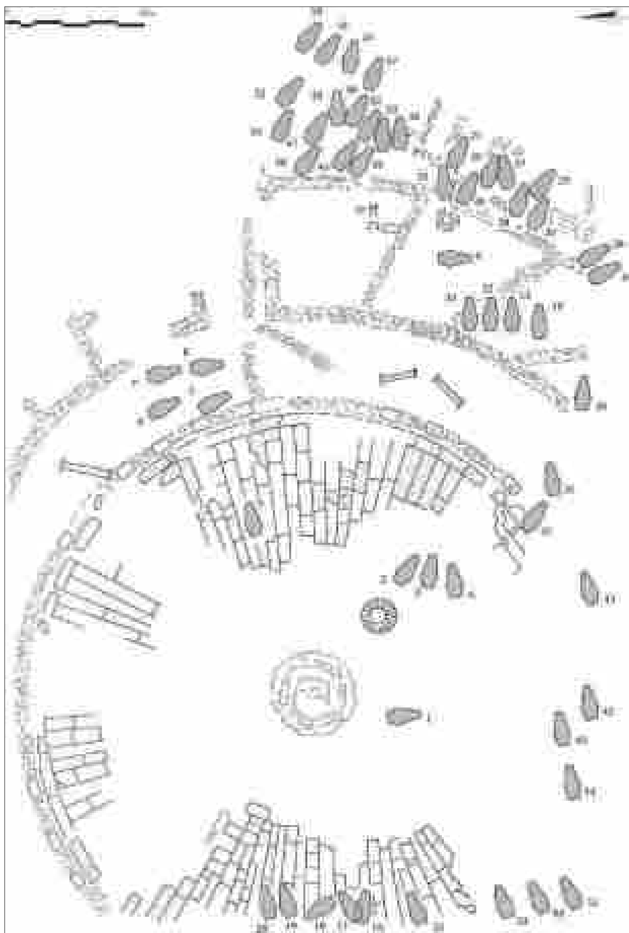
Fig. 5.4.3: Macellum-forum . Planimetria schematica dell'edificio con indicate le sepolture rinvenute nell'area (rielaborazione grafica da HOTI et alii 2008, p. 373, fig. 4).
