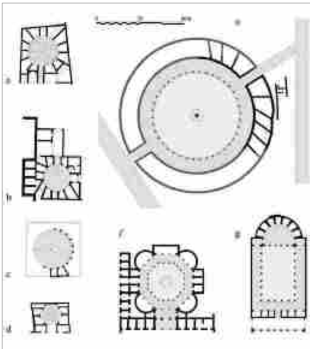
Fig. 5.4.33. Tavola comparativa con la pianta del macellum/forum rapportata a quella di altri macella di età imperiale: a) Herdonia ; b) Alba Fucens ; c) Aclanum ; d) Saepinum ; e) Durazzo: macellum/forum ; f) Gerasa ; g) Timgad (disegno P. Baronio).
