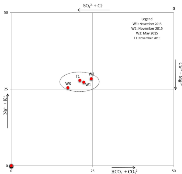
Fig. 7. Chebotarev diagram.
