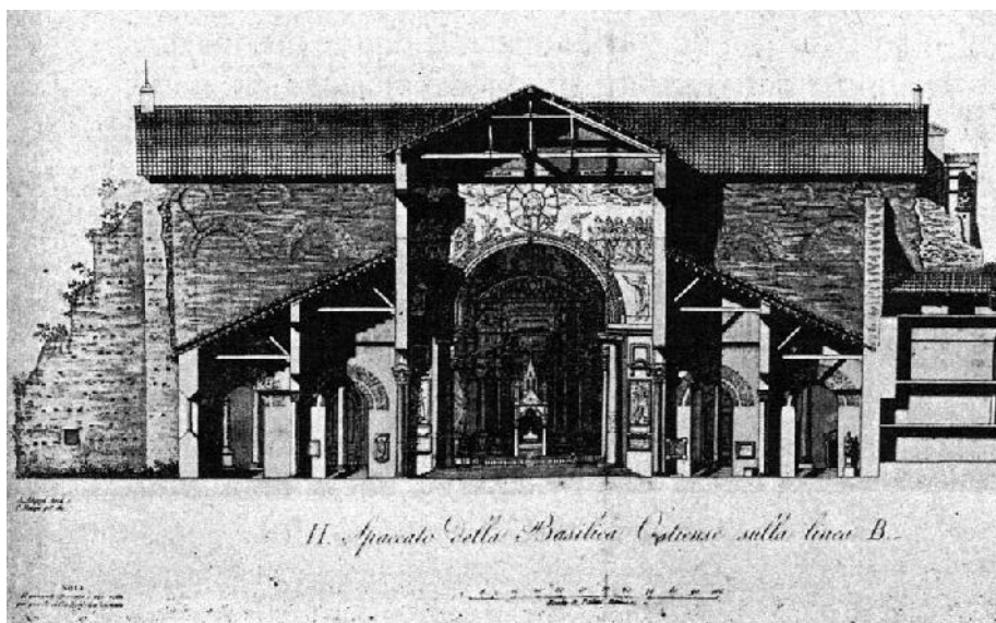
Fig. 12 - S. Paolo fuori le mura. Andrea Alippi, sezione trasversale delle navate, prima dell'incendio del 1823. (da Nicola Maria Nicolai, Della basilica di S. Paolo , Roma, 1815)
