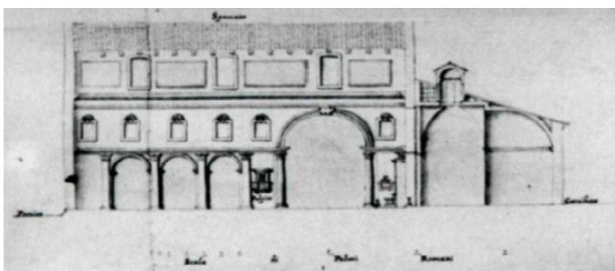
Fig. 14 – SS. XII Apostoli, sezione. (da Lorenzo Finocchi Ghersi, La Basilica dei SS. Apostoli , Roma, 1991)
