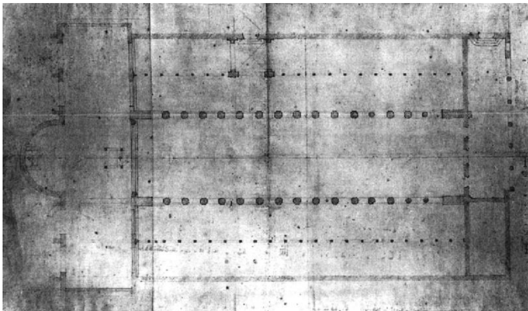
Fig. 5 - Francesco Borromini, Rilievo dell'antica basilica di San Giovanni in Laterano. (Vienna, Albertina, Az Rom 374, da A. Roca De Amicis, L'opera di Borromini in S. Giovanni in Laterano , Roma, 1995)
