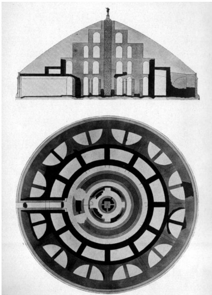
Fig. 43 – A.M. Colini, G. Gatti, G. Q. Giglioli, Ricostruzione grafica in pianta e sezione del Mausoleo. (da Il Mausoleo di Augusto in “Capitolium”, n.10, ottobre 1930)
