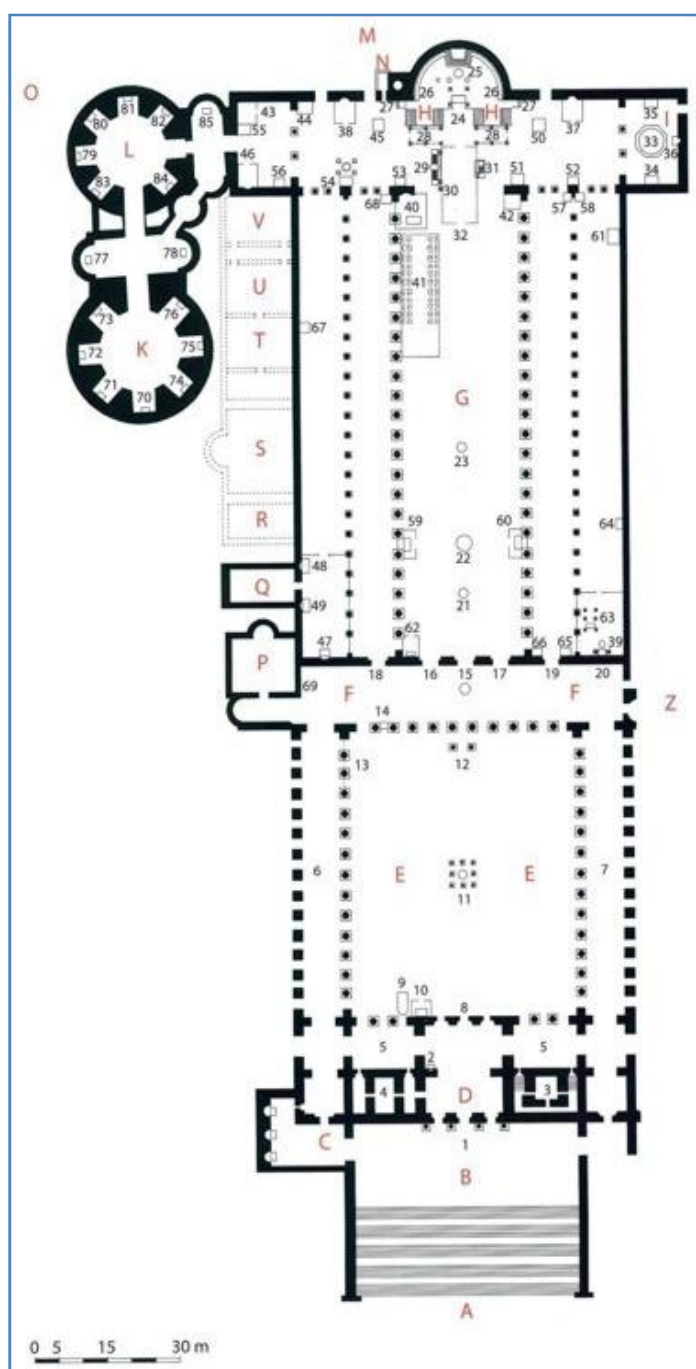
Fig. 27 - Pianta della Basilica di S. Pietro in Vaticano (secoli VI-XV). (Elaborazione da Alfarano, 1590 e De Blaauw, 1994)
