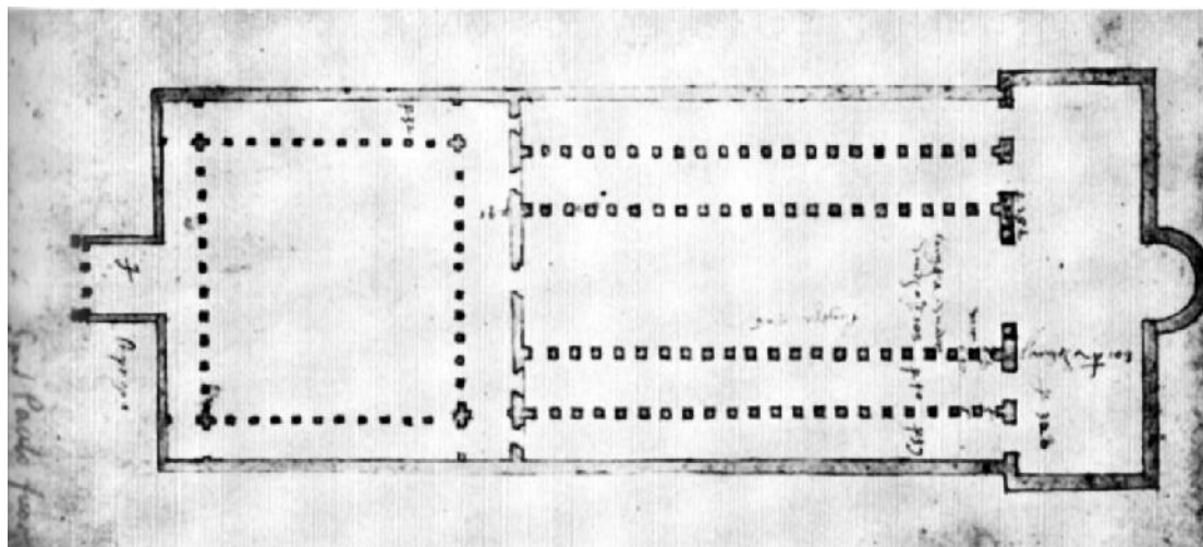
Fig. 10 - San Paolo fuori le mura. Anonimo, Pianta della basilica e dell'atrio, 1490-1510 ca., (Vienna, Albertina IT AZ 703, da Richard Krautheimer, Corpus Basilicarum Christianarum Romae , Città del Vaticano, 1937).
